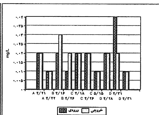
نمودار ۱۱. تغییرات غلظت مس در آب ورودی و خروجی مزارع
