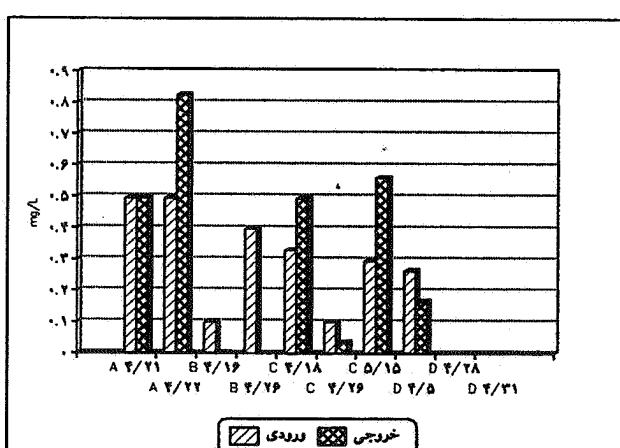
نمودار ۱۳. تغییرات غلظت NO_3 در آب ورودی و خروجی مزارع
