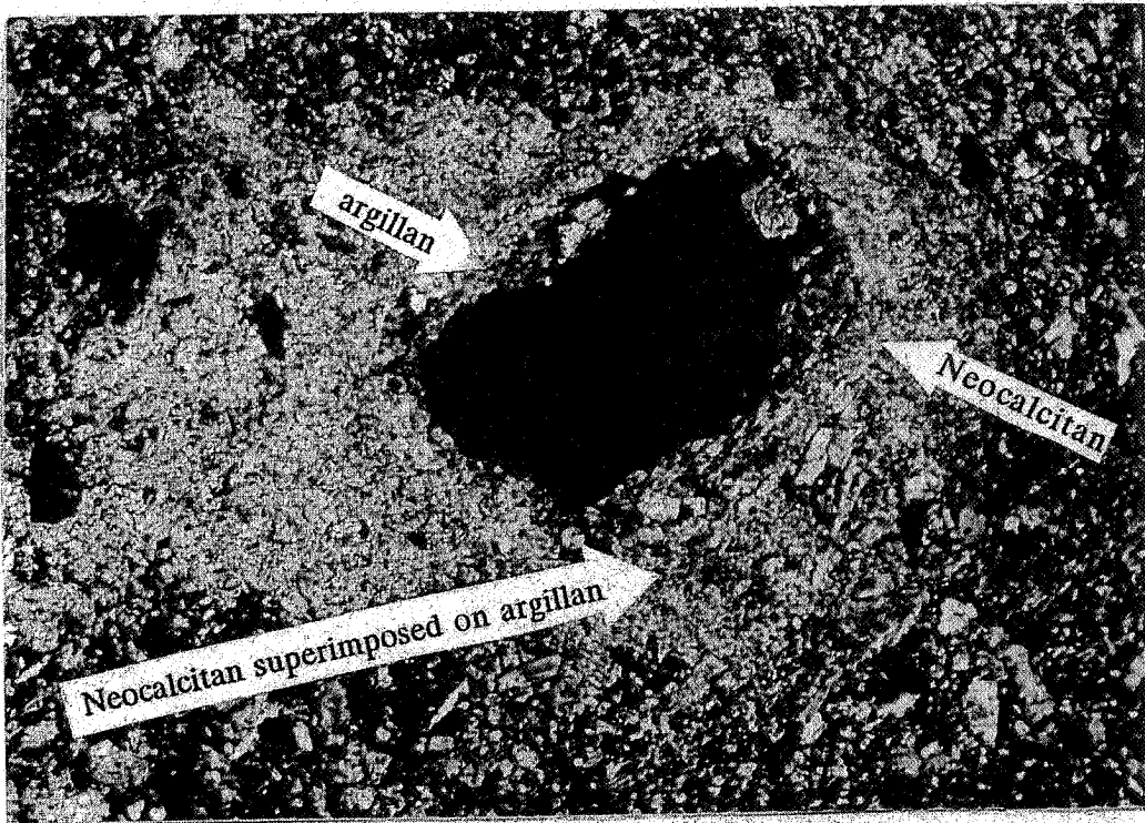
شکل ۹. مقطع میکروسکوپی افق Btk پروفیل ۸، نور پلاریزه، طول عکس برابر ۰/۵ میلی متر (نئوکلستیان روی آرگیلان و تخریب بخشی از آرگیلان را نشان می دهد).
