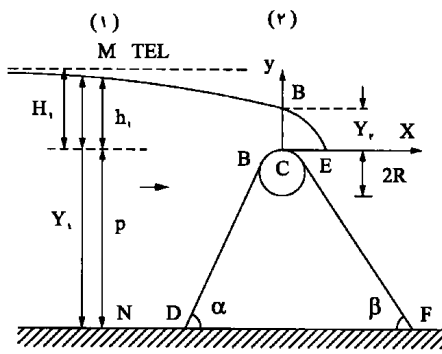
شکل ۱. جریان عبوری از روی یک سرریز تاج دایره‌ای
