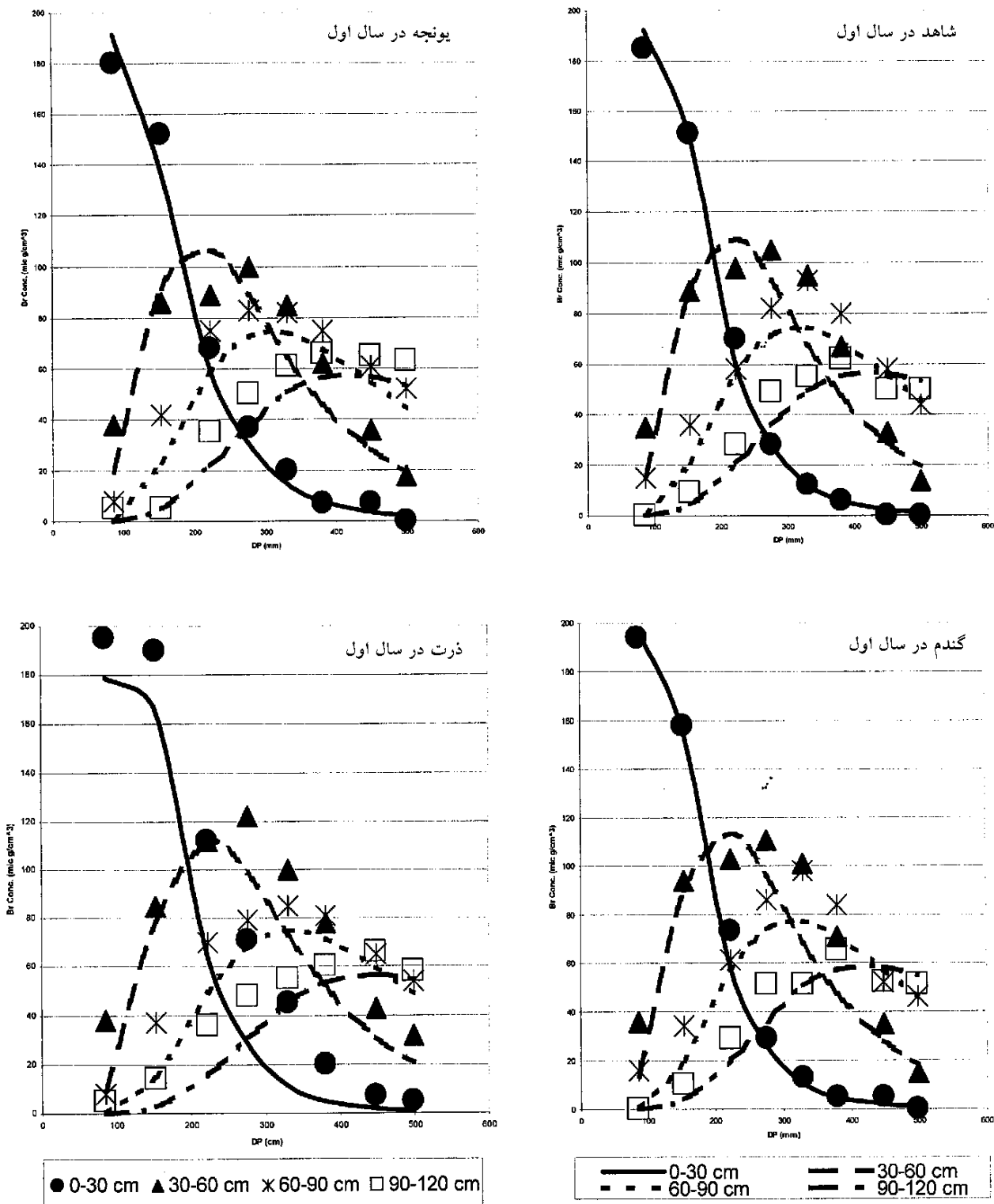
شکل ۱. غلظت‌های اندازه‌گیری شده (نشانه‌ها) و مقادیر برازش شده (خطوط) به وسیله مدل RSM در سال اول. محور افقی نمودارها مقدار نفوذ عمقی (DP) بر حسب میلی‌متر و محور عمودی غلظت برمایند بر حسب میکروگرم بر سانتی‌متر مکعب خاک است.
