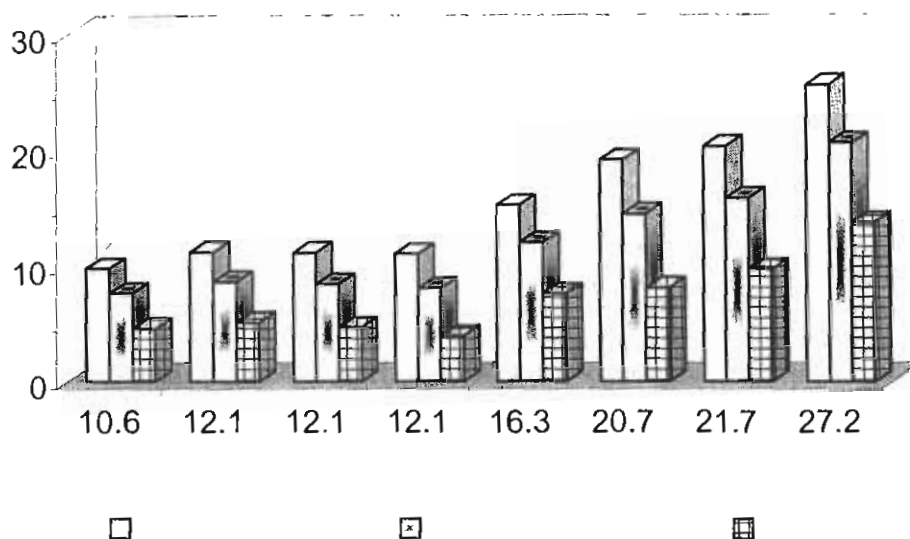
شکل ۳. مقادیر عمق بهینه به ازای میانگین های مختلف پخش آب از دستگاه در مدیریت های مختلف آبیاری، روش نرمال
