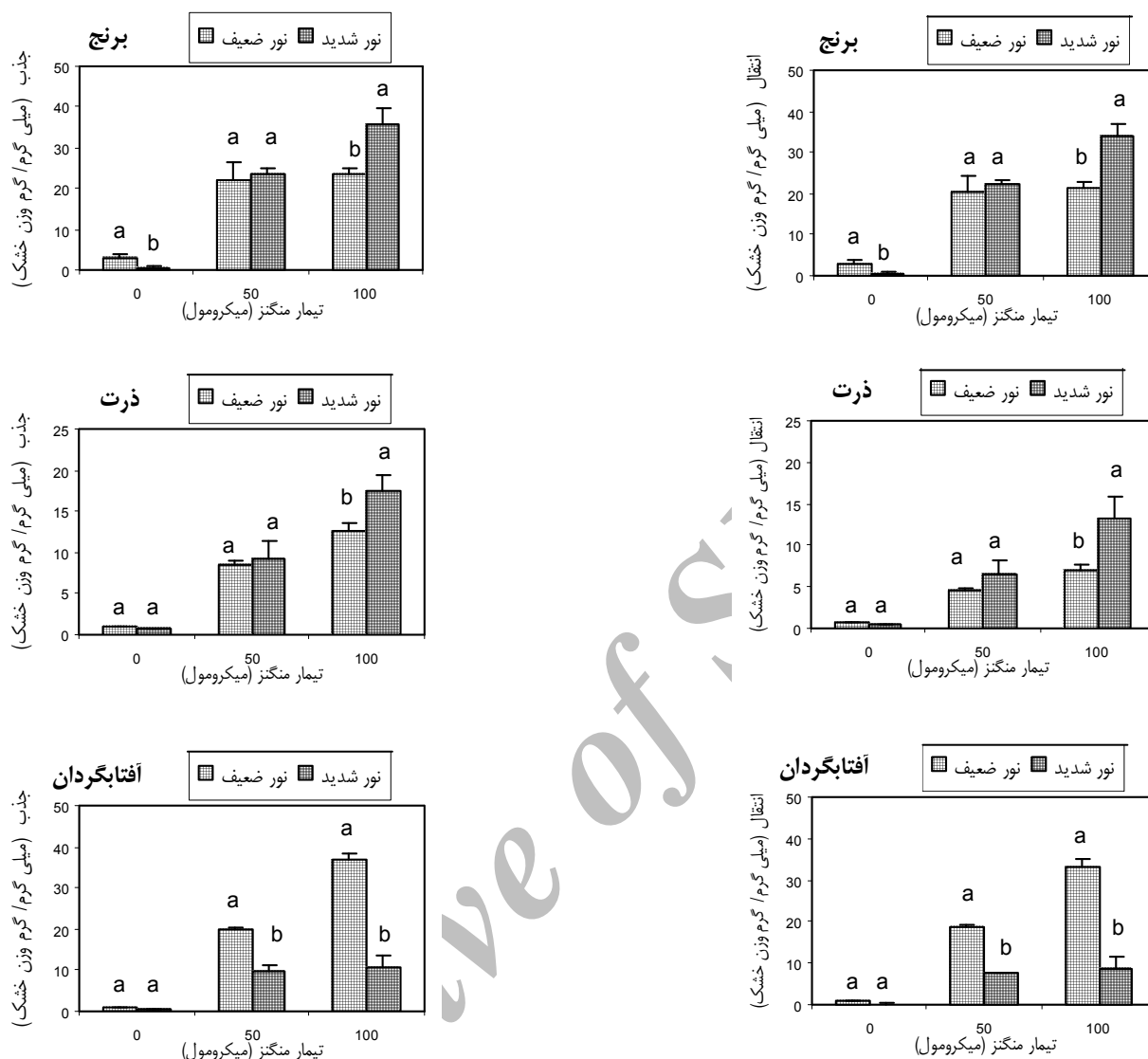
شکل ۲. جذب ( \text{mg g}^{-1}\text{RDW} ) و انتقال ( \text{mg g}^{-1}\text{RDW} ) منگنز در سه گیاه برنج، ذرت و آفتابگردان که در شرایط نوری مختلف (نور ضعیف و نور شدید) و در غلظت‌های مختلف مسموم کننده منگنز رشد کرده‌اند. زوج ستون‌هایی که با حروف یکسانی مشخص شده‌اند، فاقد تفاوت معنی‌دار بوده‌اند ( P < 0.05 )
