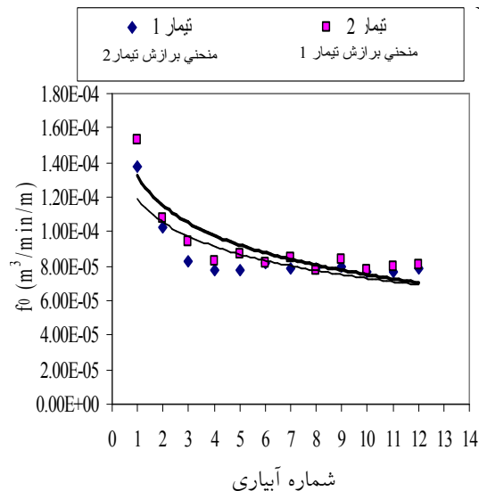
شکل ۷. تغییرات مقادیر ضریب f₀ در تیمارهای ۱ و ۲ در آبیاری‌های متوالی در طی یک فصل رشد
