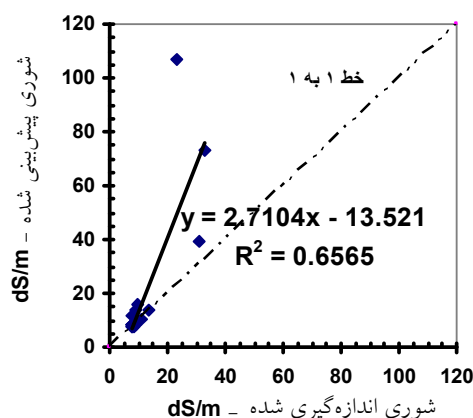
شکل ۳. مقایسه مقادیر اندازه‌گیری شده شوری در برابر مقادیر پیش‌بینی شده با مدل SWAP (بالاچپ) LEACHC (بالا راست) و معادله ۱ (پایین) در تیمار D1L1
