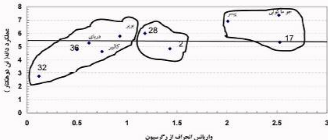
شکل ۳. پراکنش ژنوتیپ‌ها بر مبنای میانگین عملکرد دانه و مقادیر انحراف از رگسیون خطی، (پارامتر دوم ابرهات و راسل) خطوط به هم پیوسته گروه‌بندی‌های حاصل از تجزیه خوشه‌ای بر مبنای واریانس انحراف از رگسیون را نشان می‌دهند و خط افقی ممتد از میانگین عملکرد دانه می‌گذرد.
