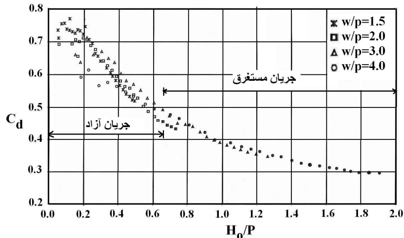
شکل ۳. ضریب جریان ( C_d ) به صورت تابعی از H_0/P و W/P به ازای (R/w = 0/15) - آزمون (W3-Ri)
