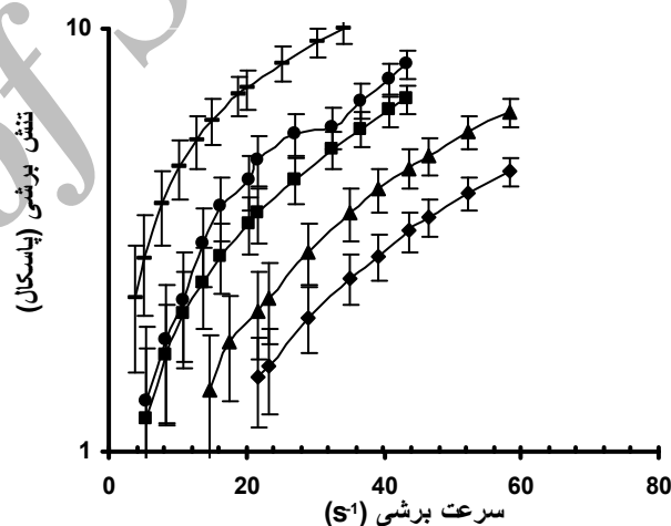
شکل ۳. نمایش تغییرات سرعت برشی در مقابل تنش برشی در محلول‌های پودر ثعلب در غلظت‌های مختلف (۷، ۶، ۵، ۴، ۳، ۲٫۵ گرم در لیتر) در دمای ۲۵ درجه سانتی‌گراد و پ هاش ۷.
