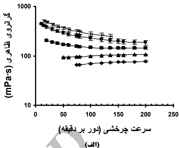
شکل ۲. نمایش رفتار جریان محلول‌های پودر ثعلب در غلظت‌های مختلف (۷، ۶، ۵، ۴، ۳، ۲٫۵ گرم در لیتر) در دمای ۲۵ درجه سانتی‌گراد و پ هاش ۷ (الف) سرعت چرخشی در مقابل گرانیوی ظاهری (ب) سرعت برشی در مقابل گرانیوی ظاهری.
