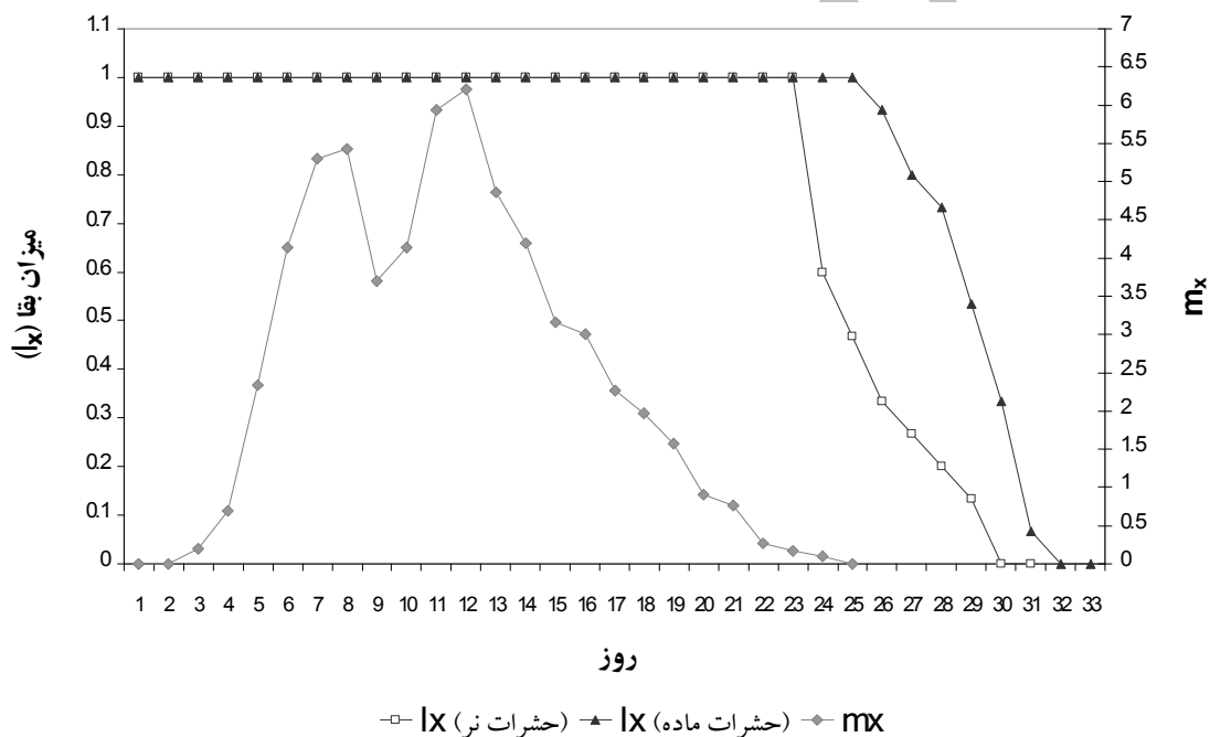
شکل ۱. تعداد افراد ماده تولید شده در روز از هر فرد ماده ( m_x ) و میزان بقای حشرات کامل نر و ماده ( l_x ) در طول دوره پس از خروج
