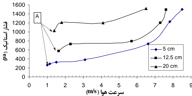
شکل ۲. منحنی مشخصه افت فشار- سرعت هوا برای شرایط بستر سیال در عمق های ۵ cm، ۱۲/۵ cm و ۲۰ cm (A= نقطه حداقل سیال سازی)
