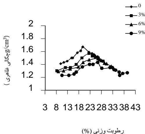
شکل ۸. اثر سطوح مختلف تفاله پسته بر منحنی تراکم خاک لوام رسی سیلتی
