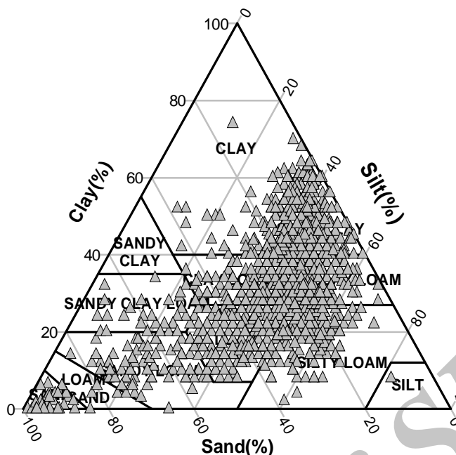
شکل ۳. نمایش توزیع اندازه ذرات معدنی خاک برای مجموع داده‌ها در نمودار مثلث بافت خاک آمریکا
