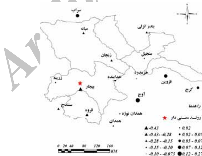
شکل ۴. وضعیت روند مجموع بارش سالانه برای ایستگاه‌های سینوپتیک منتخب حوضه آبخیز سد سفیدرود
