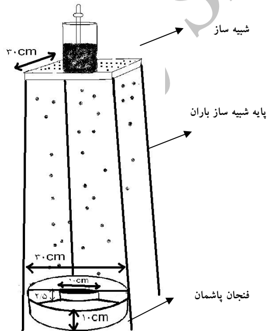
شکل ۲. نمایی از شبیه ساز باران، پایه شبیه ساز باران و فنجان پاشمان
