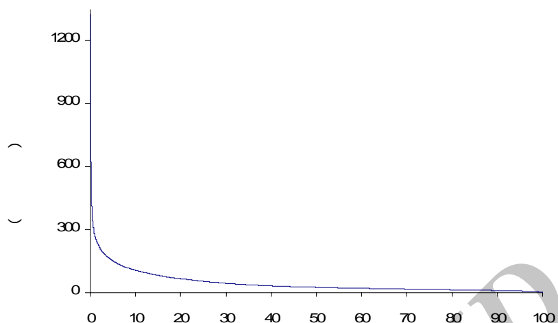
شکل ۲. منحنی تداوم جریان در ایستگاه آفرینه
