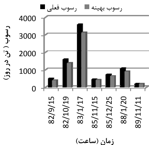
شکل ۸. مقایسه رسوب کاربری فعلی و بهینه کاربری اراضی
