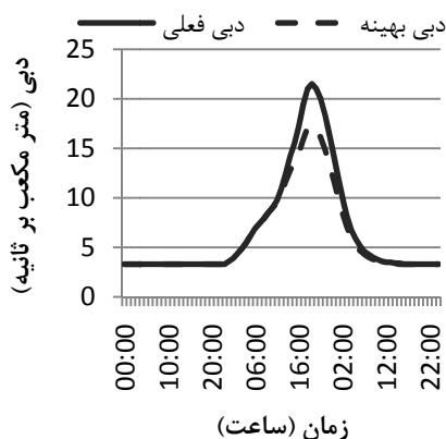
شکل ۷. مقایسه هیدروگراف شبیه‌سازی در شرایط کاربری
