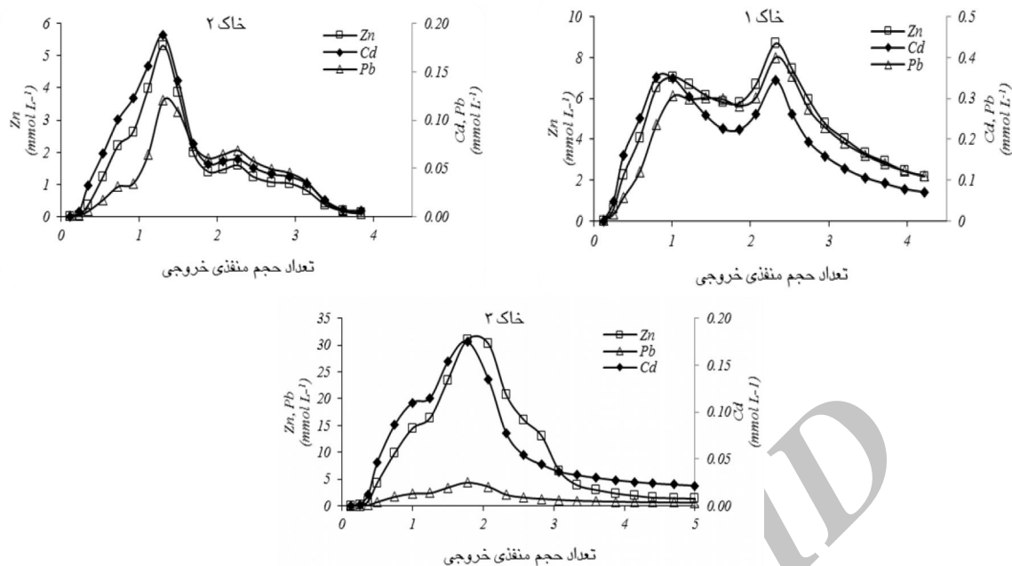
شکل ۸. تغییرات غلظت Zn، Cd و Pb با محلول ۰/۲ مولار EDTA (در محلول زمینه ۰/۱ مولار نیترات کلسیم) در روش ستونی پالسی در سه خاک
