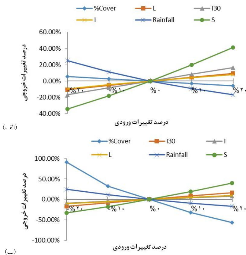
شکل ۵. نمودارهای آنالیز حساسیت، (الف) شیب ۶۰ درصد و (ب) شیب کمتر از ۶۰ درصد
