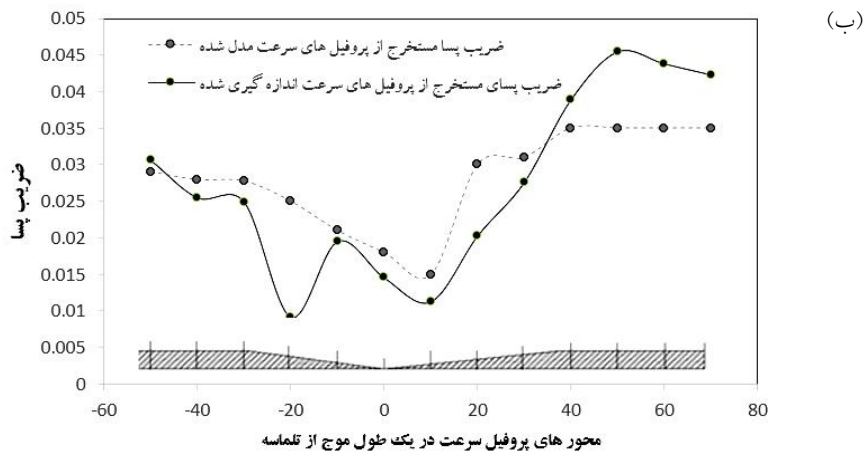
شکل ۵. نمایش ضریب پسا برای ذرات مستقر بر الف) تلماسه تاج تخت و ب) تاج تیز در شرایط هیدرولیکی دبی ۳۰ لیتر بر ثانیه و عمق ۳۲ سانتی‌متر
