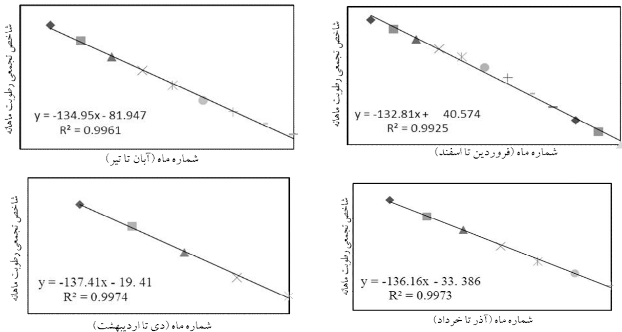
شکل ۱. نمودار شاخص رطوبت تجمعی ماهانه و خط برازش شاخص ایستگاه بندرانزلی با دوره‌های ارزیابی متفاوت (خیلی مرطوب معتدل)
