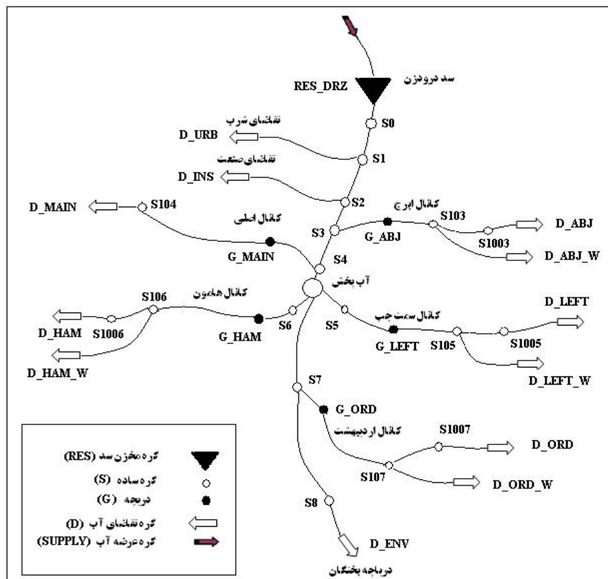
شکل ۱. نمای شماتیک شبکه آبیاری سد درودزن
