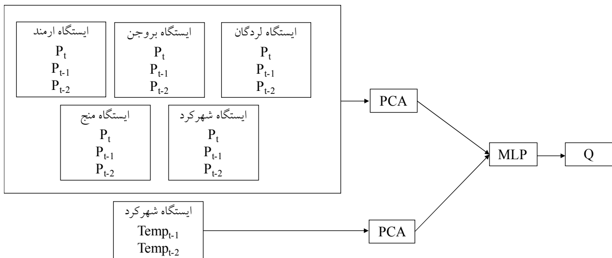
شکل ۲. روند مدل‌سازی بارش - رواناب در تحقیق حاضر
