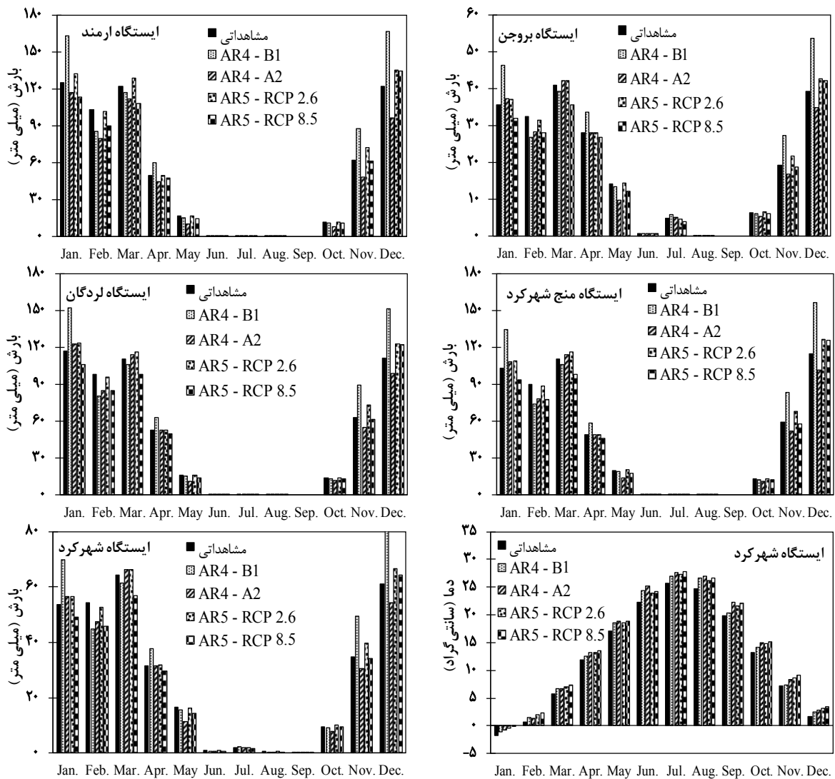
شکل ۳. مقایسه متوسط بارش ماهانه در دوره پایه ۲۰۰۰-۱۹۷۱ و دروه آتی ۲۰۲۱-۲۰۵۰ در ایستگاه‌های مورد مطالعه
