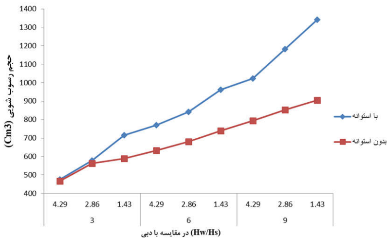
شکل ۱۴. نمودار تأثیر نیم استوانه بر حجم رسوب شویی
