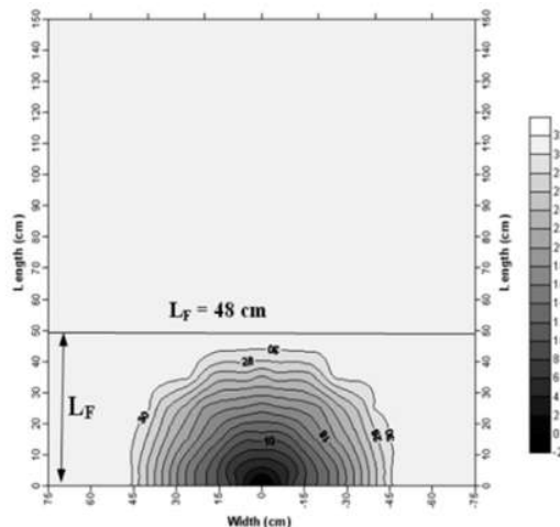
شکل ۶. توپوگرافی بستر مخروط رسوب شویی (رسوبات درشت دانه)
