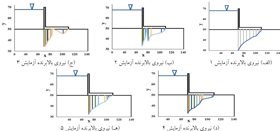
شکل ۷. برآورد نیروی بالابرنده در مدل‌ها
