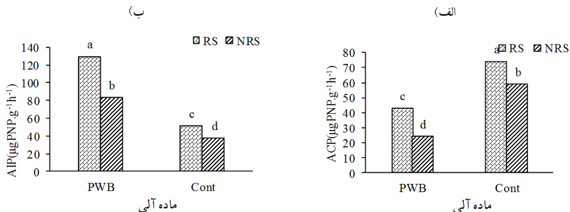
شکل ۳. مقایسه میانگین اثر متقابل ماده آلی و خاک بر فعالیت آنزیم‌های فسفاتاز اسیدی و قلیایی ACP و ALP ، RS ، Cont ، PWB و NRS به ترتیب آنزیم‌های فسفاتاز اسیدی، قلیایی، بیوجار ضایعات هرس، شاهد بدون ماده آلی، خاک ریزوسفر و غیر ریزوسفر
