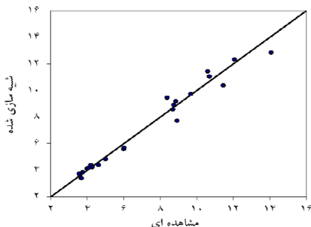
شکل ۶. همبستگی مقادیر شوری خاک شبه‌سازی شده و مشاهده‌ای در ناحیه ریشه (dS/m)
