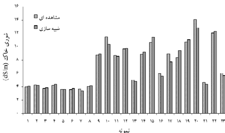
شکل ۷. مقادیر شوری خاک شبه‌سازی شده و مشاهده‌ای در مزرعه چغندر قند
