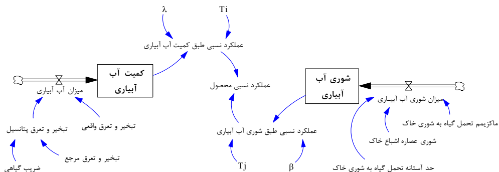
شکل ۳. نمودار حالت و جریان عملکرد محصول (۲)
