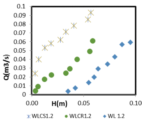
شکل ۱۰. تأثیر کنگره‌های جدید در WLCR
