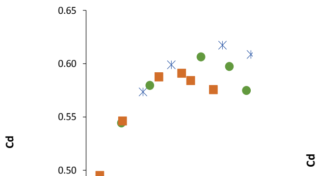
شکل ۸. مقایسه ضرایب دبی نسبت به H_t/p با ارتفاع ۱۵ سانتی متر
