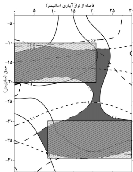
شکل ۶. هم‌پوشانی منحنی‌های رطوبت نسبی خاک در محدوده (0.9 < \theta_{avg} < 1.1) و (0.7 < \theta_{avg} < 0.9) روز پس از کاشت
