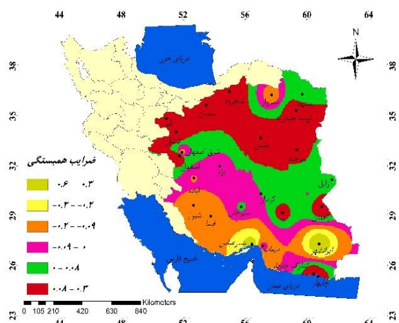
شکل ۴. پهنه بندی ضریب همبستگی متغیر میانگین دما با فراوانی وقوع طوفان‌های گردوغبار در فصل تابستان
