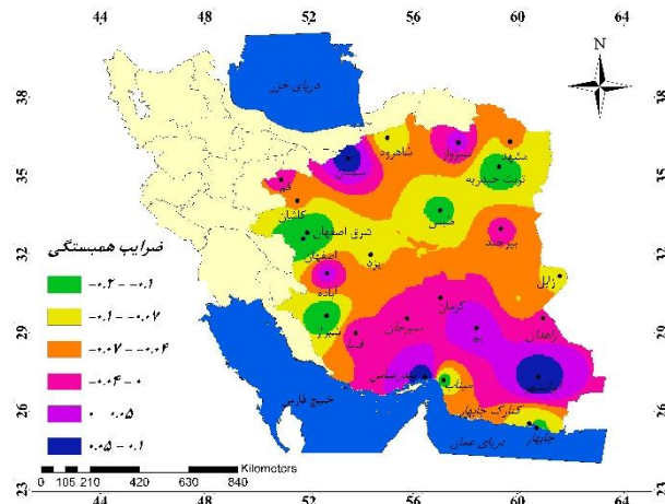
شکل ۷. پهنه بندی ضریب همبستگی متغیر میانگین بارش با فراوانی وقوع طوفان‌های گردوغبار در فصل تابستان
