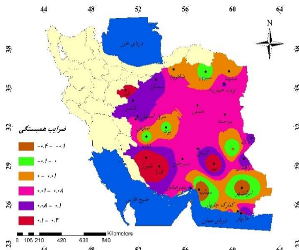
شکل ۳. پهنه بندی ضریب همبستگی متغیر بیشینه دما با فراوانی وقوع طوفان‌های گردوغبار در فصل تابستان
