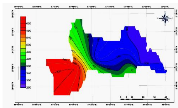
شکل ۲۰. توزیع TDS در حوضه هلیلرود در سال ۱۳۷۴
