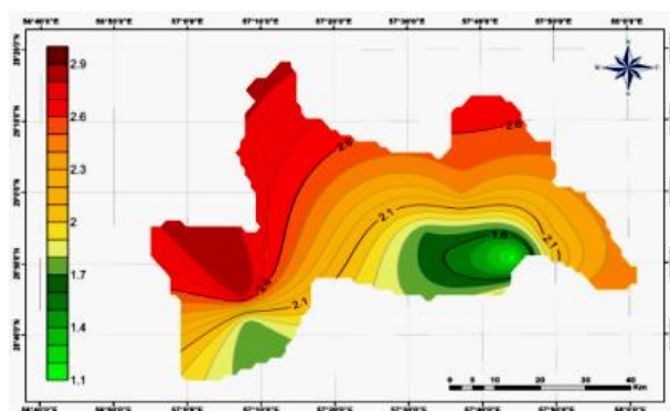
شکل ۲. نقشه پهنه‌بندی SPI سال ۱۳۷۴
