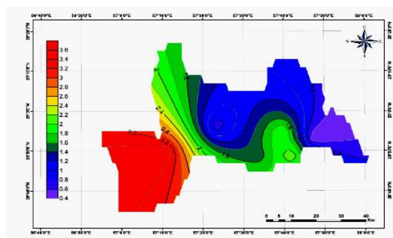
شکل ۲۲. توزیع SAR در حوضه هلیلرود در سال ۱۳۷۴
