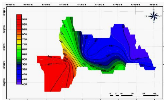
شکل ۱۸. توزیع EC در حوضه هلیلرود در سال ۱۳۷۴
