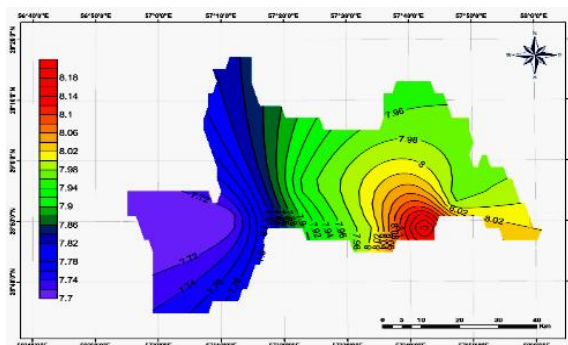
شکل ۱۶. توزیع pH در حوضه هلیلرود در سال ۱۳۷۴
