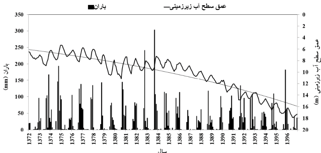
شکل ۳. هیدروگراف واحد آبخوان دشت شیراز
