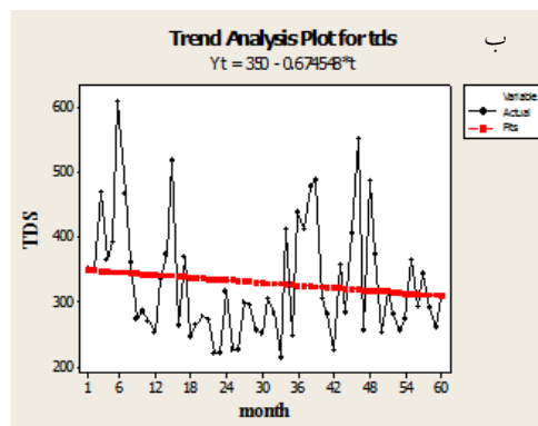
شکل ۵. الف) نقشه تغییرات مکانی و ب) روند تغییرات پنج‌ساله کل نمک‌های محلول در آب (میلی‌گرم در لیتر)
