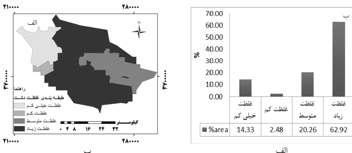
شکل ۱۰. الف) نقشه تلفیقی لایه‌های مختلف کیفی دشت خرم‌آباد و ب) نمودار درصد غلظت‌های مختلف دشت
