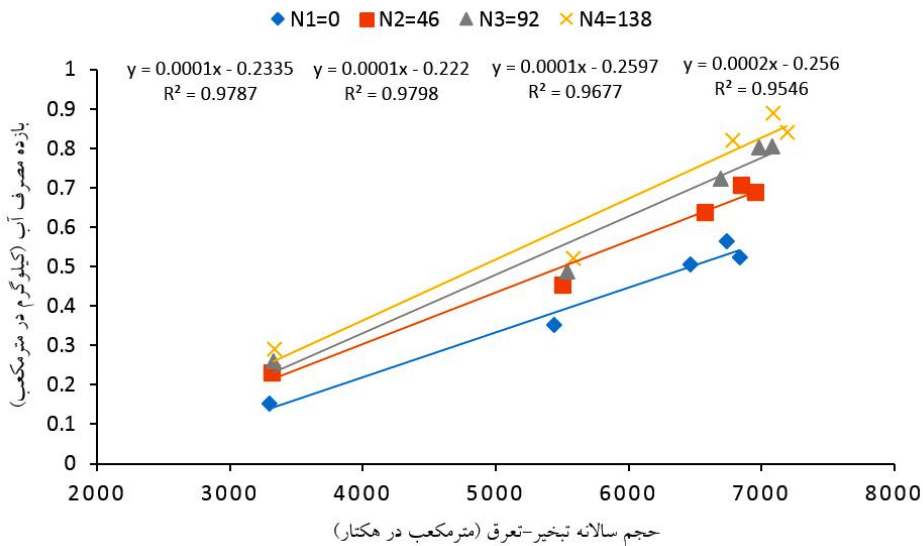
شکل ۵. رابطه بین بازده مصرف آب و مقادیر مختلف تبخیر-تعرق واقعی در مقادیر مختلف نیتروژن کاربردی
