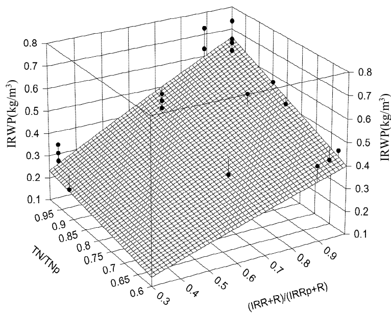
شکل ۱۰. واسنجی رابطه بین بهره‌وری آب مجموع آب آبیاری و بارندگی و مجموع آب آبیاری و بارندگی نسبی و نیتروژن نسبی موجود در ناحیه ریشه با استفاده از داده‌های سال ۱۳۸۸-۱۳۸۹
