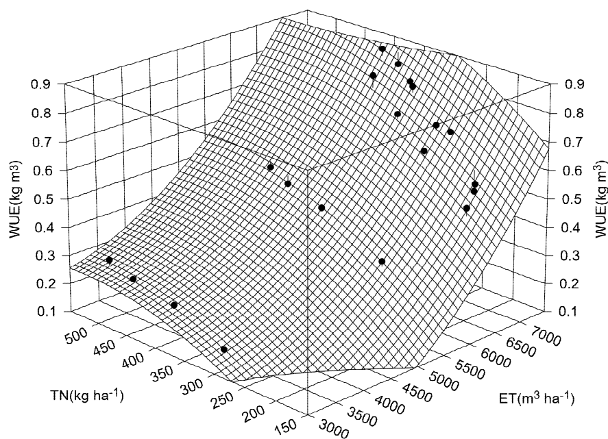
شکل ۷. واسنجی رابطه بین بازده مصرف آب، تبخیر-تعرق و مقدار کل نیتروژن موجود در خاک با استفاده از داده‌های سال ۱۳۸۸-۱۳۸۹
