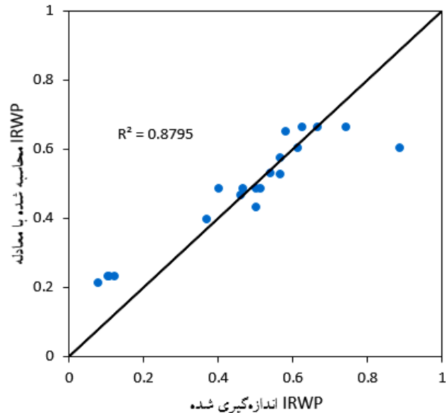
شکل ۱۲. بهره‌وری آب (IRWP) اندازه گیری و شبیه سازی شده با معادله (۸) برای سال ۱۳۸۹-۱۳۹۰
