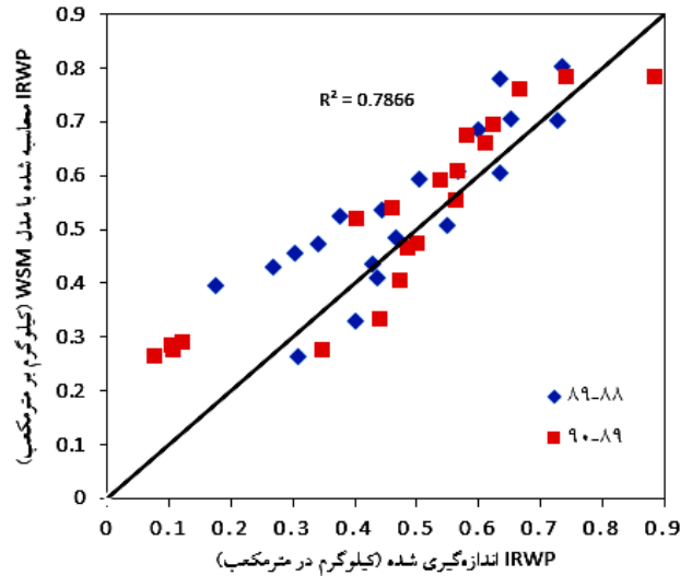
شکل ۲. بهره‌وری آب (IRWP) اندازه‌گیری و شبیه‌سازی شده با مدل WSM بر اساس مجموع آب آبیاری و باران در مقادیر مختلف نیتروژن خاک در سال‌های ۱۳۸۸-۱۳۸۹ و ۱۳۸۹-۱۳۹۰
