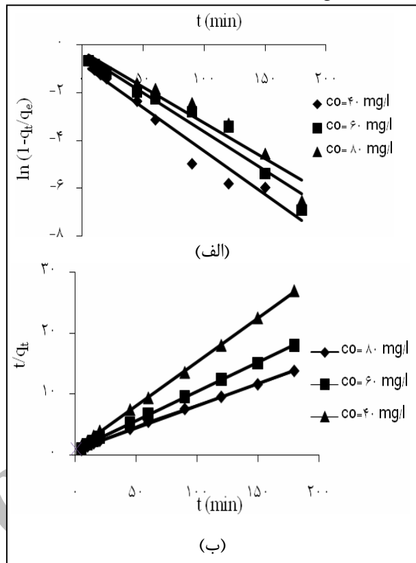
شکل ۳: نمودار خطی سینتیک شبه درجه یک (الف) و شبه درجه دو (ب) جذب کروم شش ظرفیتی بر روی خاک اره اصلاح شده درخت راجی (pH=۷) و مقدار ماده جاذب ۱۰۰g/۱۰۰cc
