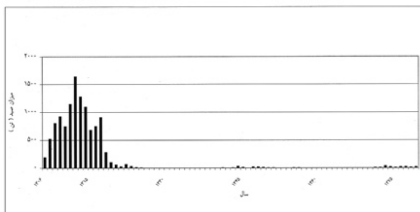
نمودار ۵: میزان صید ماهی سیم در سواحل ایرانی دریای خزر سال‌های ۱۳۰۶-۱۳۷۹
