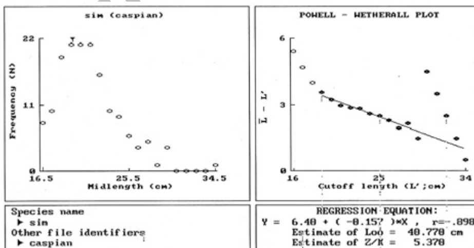
نمودار ۳: منحنی Powell - Wetherall ماهی سیم دریای خزر در سال ۱۳۸۰ - ۱۳۷۹
