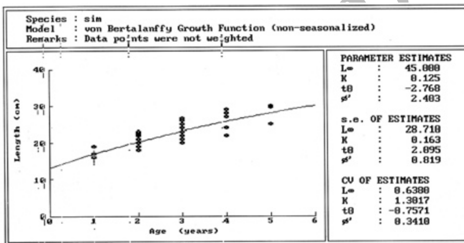
نمودار ۲: منحنی رشد بر تلافی ماهی سیم دریای خزر در سال ۱۳۸۰ - ۱۳۷۹
