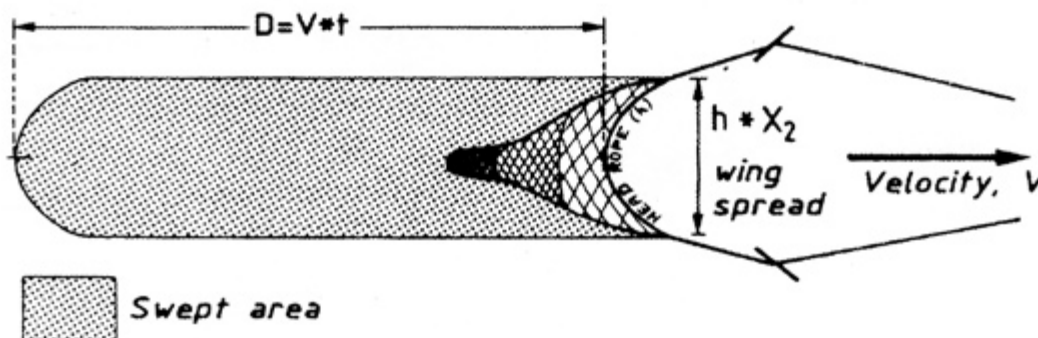
شکل ۳: مساحت جاروب شده توسط تور ترال (اقتباس از Sparre and Venema, ۱۹۹۲)
