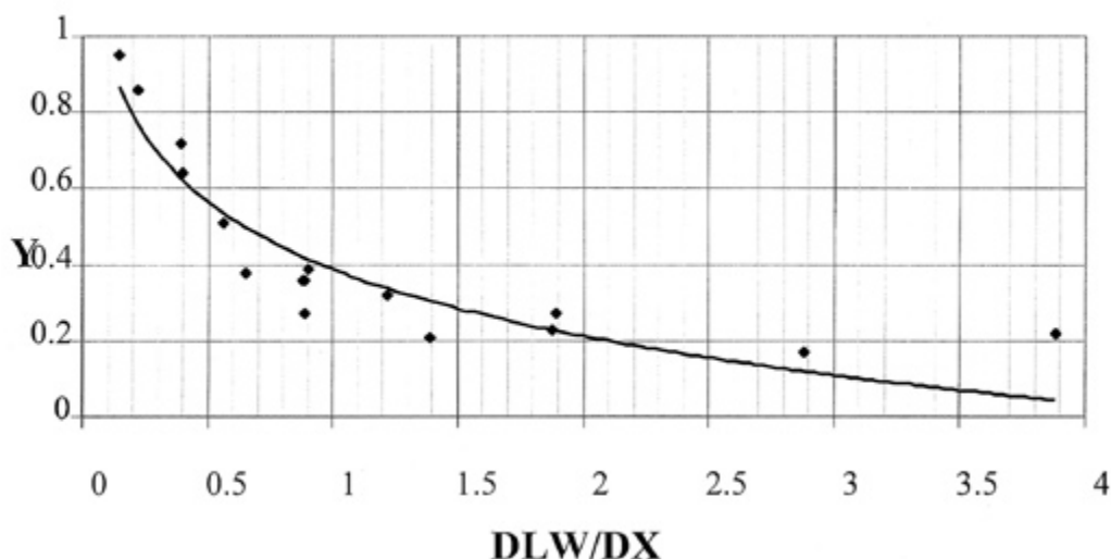
منحنی شماره ۱: منحنی شوری زدائی قسمتی از اراضی حاشیه کویر بجنستان
