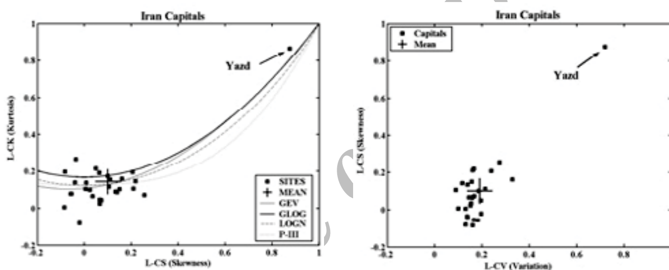
شکل ۲- نمودار گشتاورهای خطی برای ایستگاه‌های مورد مطالعه
