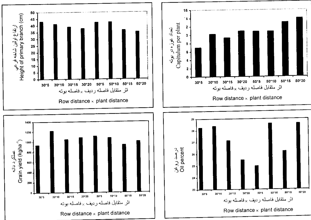
شکل ۱- نمودار اثر متقابل فاصله بین ردیف × فاصله بین بوته بر تعداد غوزه در بوته، ارتفاع اولین شاخه فرعی، درصد روغن و عملکرد دانه گلرنگ رقم اراک ۲۸۱۱
