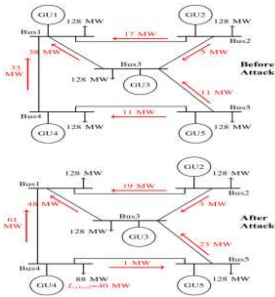
شکل ۳. توان خطوط قبل و بعد از حمله فیزیکی به واحد تولید ۱
