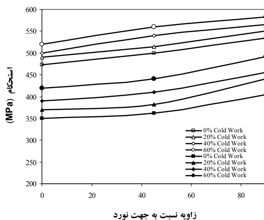
شکل ۲ تغییرات خواص کششی بر حسب زاویه نسبت به جهت نورد (علامت‌های توخالی استحکام نهایی و علامت‌های توپر استحکام تسلیم را نمایش می‌دهند)
