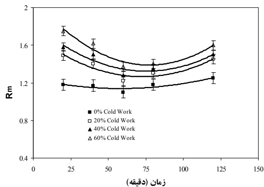
شکل ۵ پارامتر ناهمسانگردی R_m بر حسب زمان در دمای ثابت 580^\circ C به صورت تابعی از درصد کارسرد
