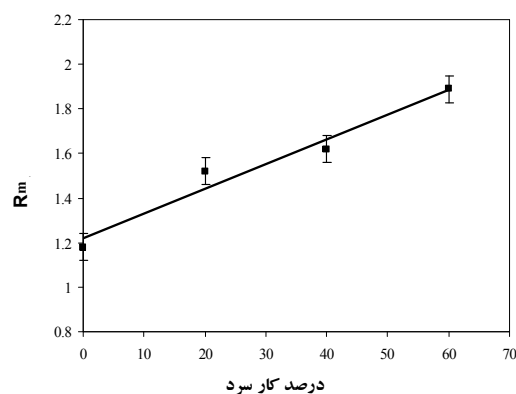
شکل ۳ نمودار تغییرات پارامتر ناهمسانگردی ( R_m ) بر حسب درصد کارسرد
