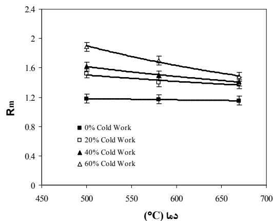
شکل ۴ نمودار تغییرات پارامتر ناهمسانگردی بر حسب دما در زمان ثابت ۴۰ دقیقه به صورت تابعی از درصد کارسرد
