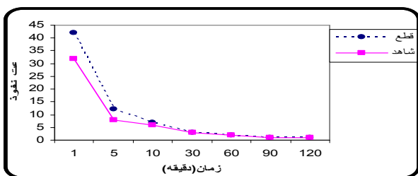
(د) مقایسه سرعت نفوذ دو قطعه پیش از عملیات
