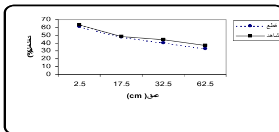
(ج) مقایسه درصد تخلخل دو قطعه پیش از عملیات
