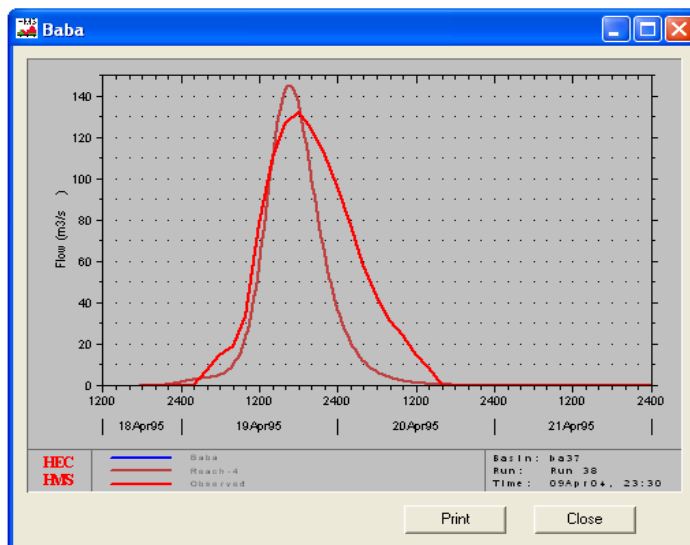
شکل ۵ - هیدروگراف شبیه‌سازی شده پس از کالیبراسیون در ایستگاه بابرود (۷۴/۱/۲۹)
