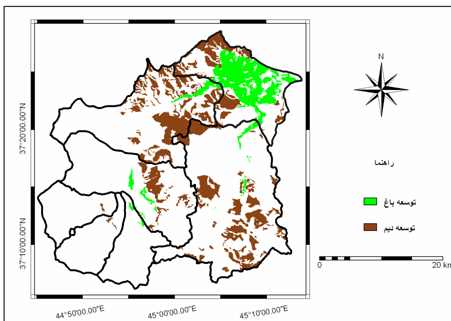
شکل ۴- نقشه توسعه اراضی دیم و باغ طی سال های ۱۳۳۴-۱۳۷۹
