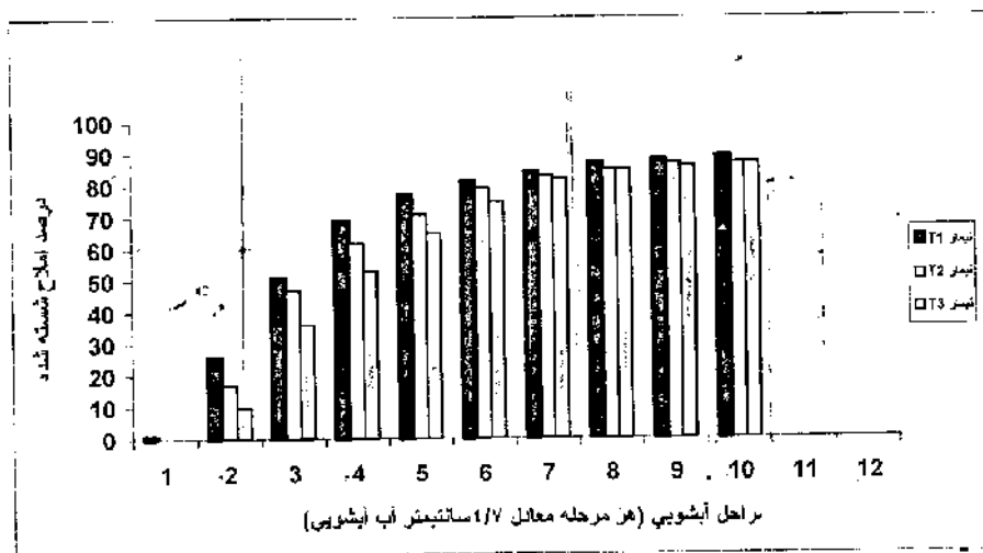
شکل (۴) درصد املاح شسته شده از عمق ۹۰ سانتیمتری خاک لکه دار برای تیمارهای مختلف
