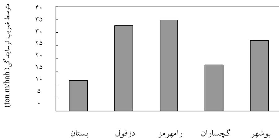
شکل ۹- تغییرات مکانی ضریب فرساینده سالانه (ton.m/ha.h) در ایستگاههای مورد مطالعه
