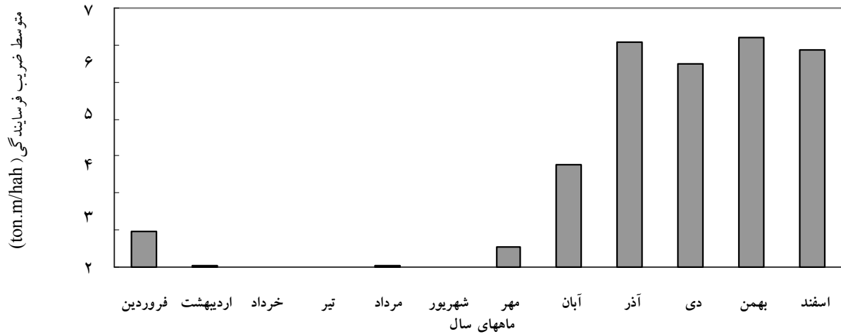
شکل ۵- تغییرات ماهانه ضریب فرسایندگی (ton.m/ha.h) در عرصه مورد مطالعه
