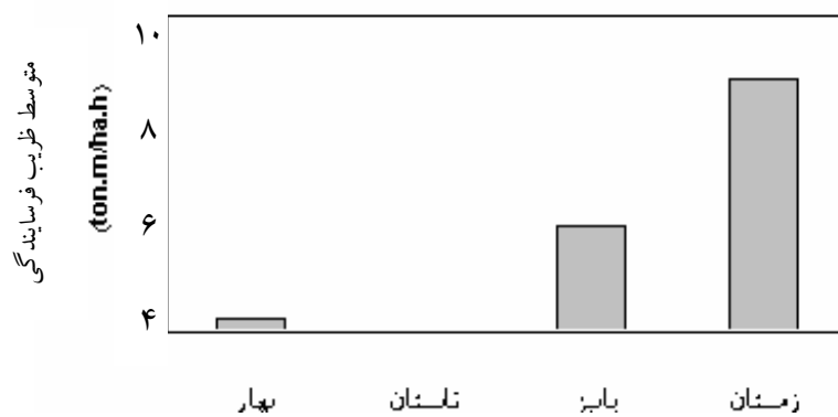
شکل ۴ - تغییرات فصلی ضریب فرسایندگی (ton.m/ha.h) در ایستگاه بستان
