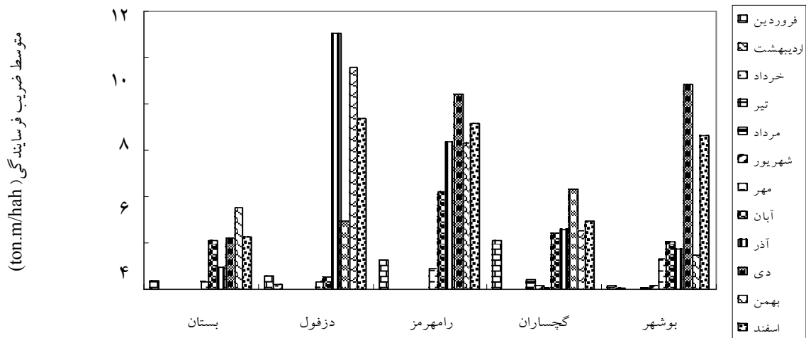
شکل ۵- تغییرات ماهانه ضریب فرسایندگی (ton.m/ha.h) در عرصه مورد مطالعه
