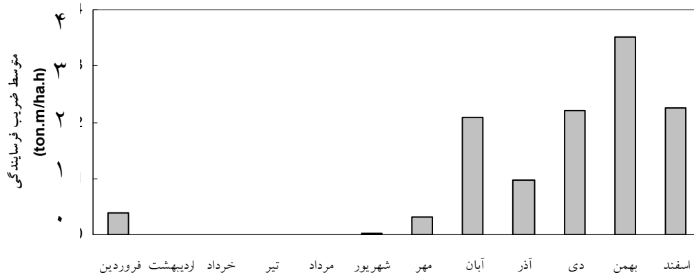
شکل ۳ - تغییرات ماهانه ضریب فرسایندگی (ton.m/ha.h) در ایستگاه بستان
