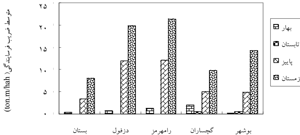
شکل ۸- تغییرات مکانی ضریب فرساینده فصلی (ton.m/ha.h) در ایستگاههای مورد مطالعه
