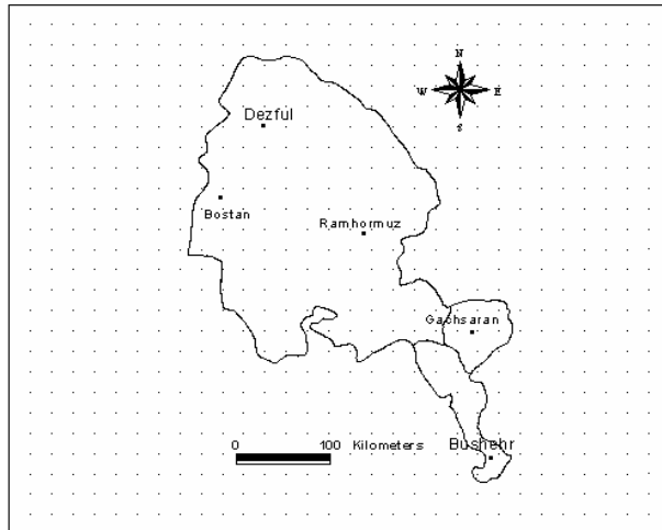
شکل ۱- نقشه پراکنش ایستگاهها در عرصه مورد مطالعه شکل ۲- نقشه تقسیمات شهری استان خوزستان استخراج پارامترهای بارندگی
