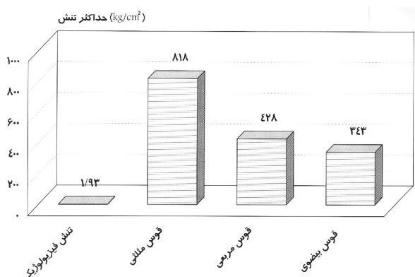
تصویر شماره ۳- حداکثر تنش در فیکسچر اول با قوسهای مربعی و بیضوی و مثلثی با تحلیل شدید استخوان
