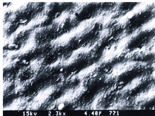
تصویر شماره ۵- سطح عاج اچ شده بعد از تابش اشعه لیزر Nd:YAG با توان ۱/۵ وات و زمان ۶۰ ثانیه
