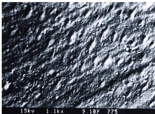
تصویر شماره ۷- سطح عاج اچ شده بعد از تابش اشعه لیزر Nd:YAG با توان ۱/۷ وات و زمان تابش ۴ ثانیه
