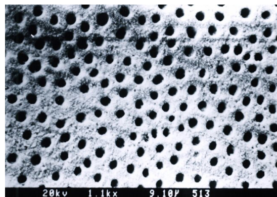
تصویر شماره ۲- عاج معمولی (همراه با لایه اسمیر) با تابش لیزر از نوع Nd:YAG با توان ۱ وات
